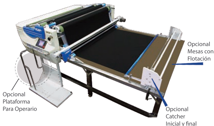
KBK-900S/ML Máquina Cortadora de banda sin fin
